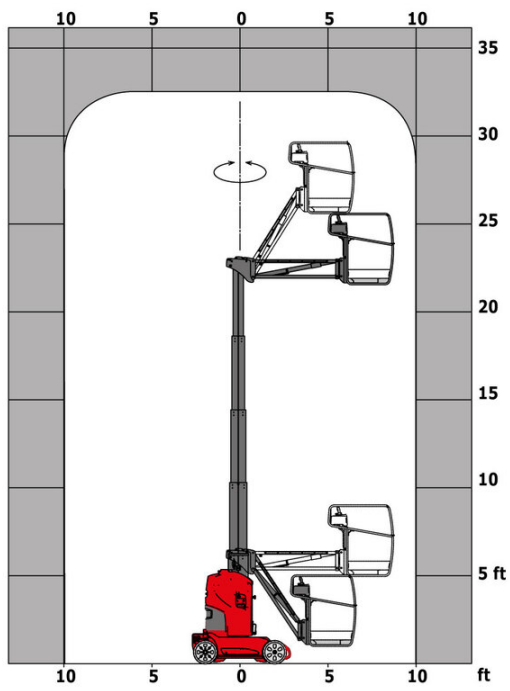
Abaque de charge pour nacelle (impérial)
