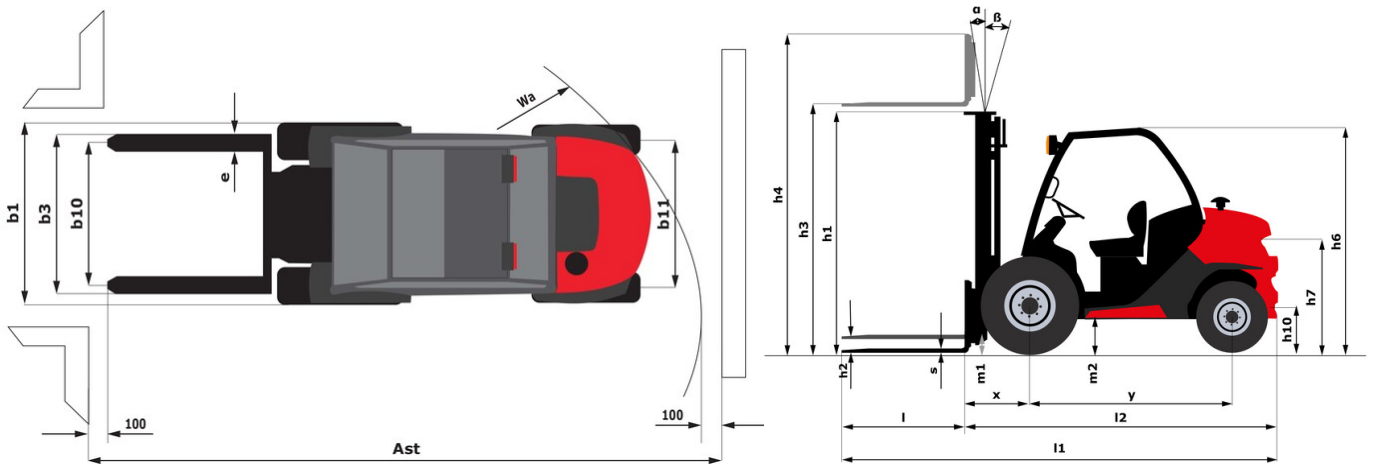
MC 25-4 ST5 - Schémas d'encombrement
