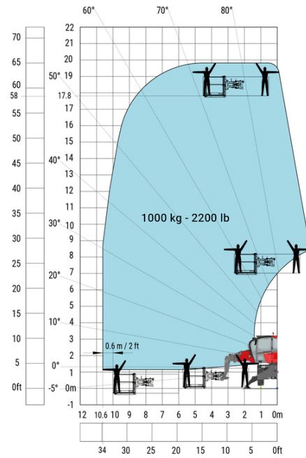
Machine sur stabilisateurs abaissés avec nacelle 1000 kg Impérial
