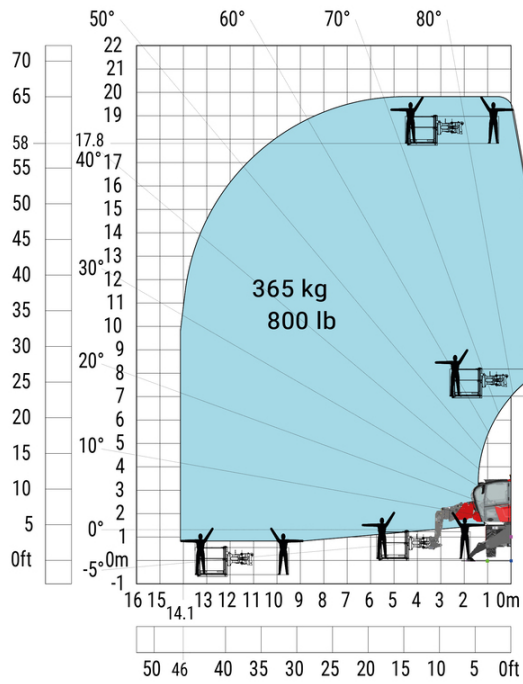
Machine sur stabilisateurs abaissés avec nacelle 365 kg
