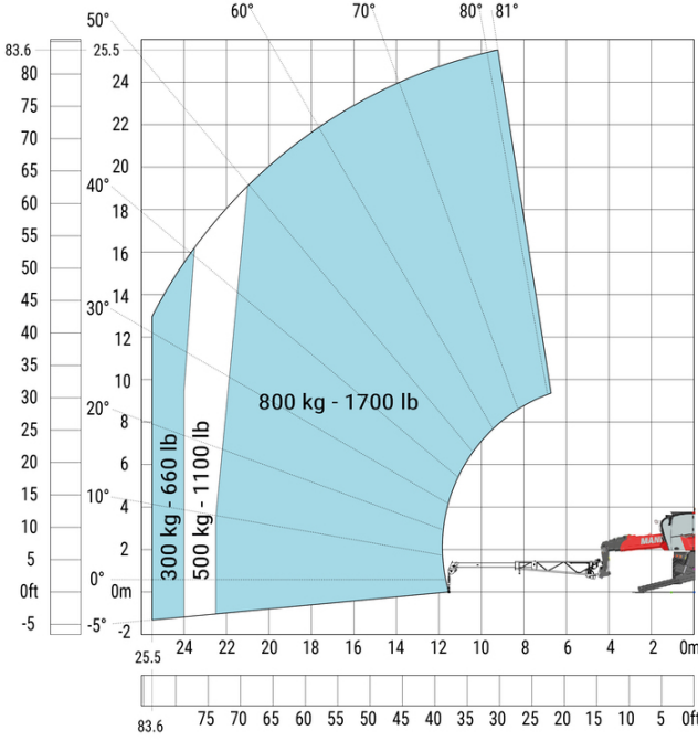
Machine sur stabilisateurs abaissés avec potence-treuil extensible (Impérial)
