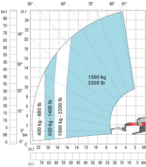
Machine sur stabilisateurs abaissés avec potence-treuil de 1500 kg (Impérial)
