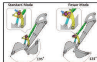
Angle de cavage ajustable
